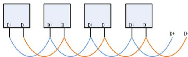
（图 2：手拉手式总线连接）
